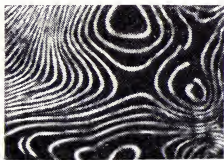
Рис. 2. Полосы равной толщины на поверхности слюдяной пластинки, характеризующие микрорельеф этой поверхности.
